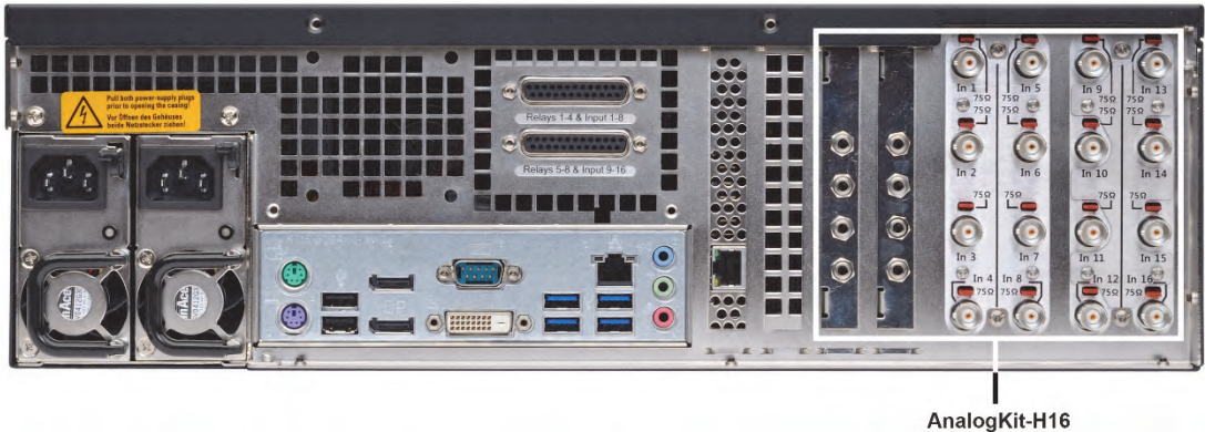
Figura 5: Conexiones de vídeo jacks BNC, Audio Line In
