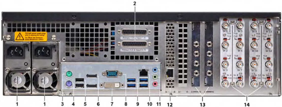
Abbildung 3: Rückansicht G-ST 6000+ G2
