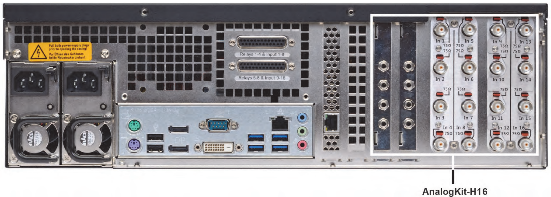
Abbildung 6: AnalogKit-H16 BNC-Eingangsbuchsen und Audio Line In
