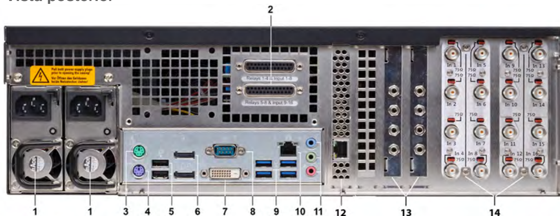
Figura 3: Vista posterior G-ST 6000+ G2
