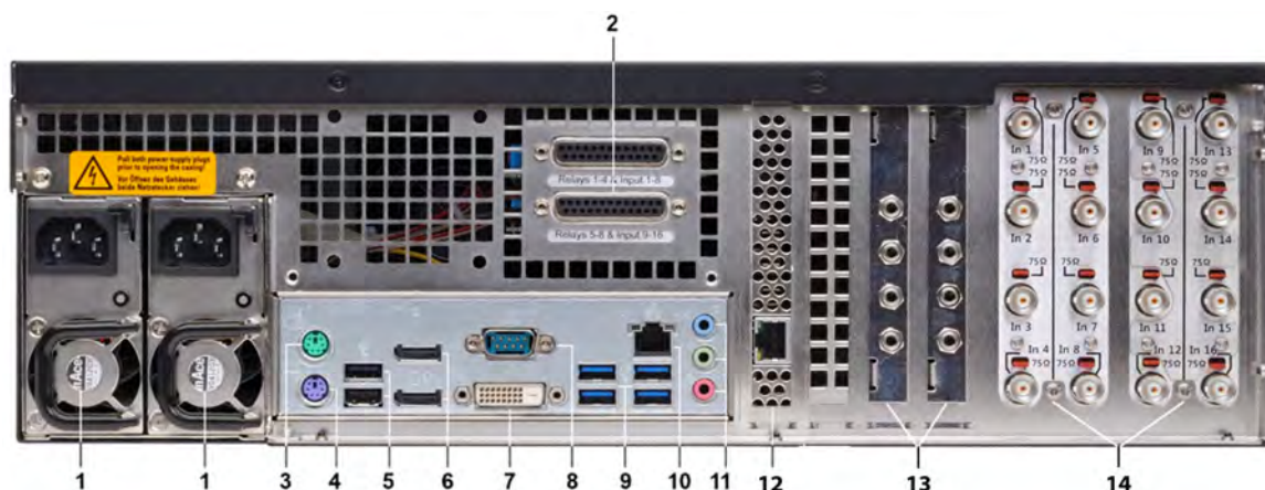
Figure 3 : vue arrière G-ST 6000+ G2
