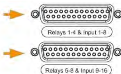
Figure 4 : prises D-Sub à 25 bornes
