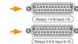
Abbildung 4: 25-polige Sub-D-Buchsen
