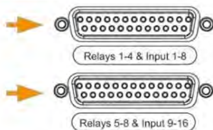
Figura 4: Zócalo Sub-D de 25 contactos
