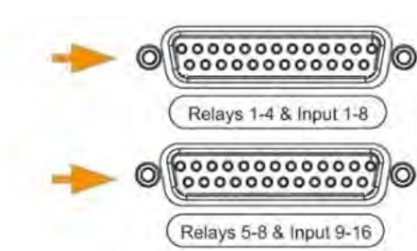
Figure 4 : prises D-Sub à 25 bornes
