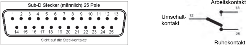
Abbildung 5: Belegung der 25-poligen Sub-D-Buchsen – lötseitig
