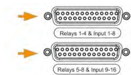
Figura 4: Zócalo Sub-D de 25 contactos
