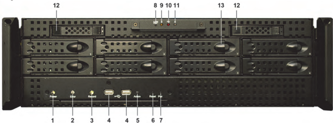
Figure 2: vue frontale sans cache
