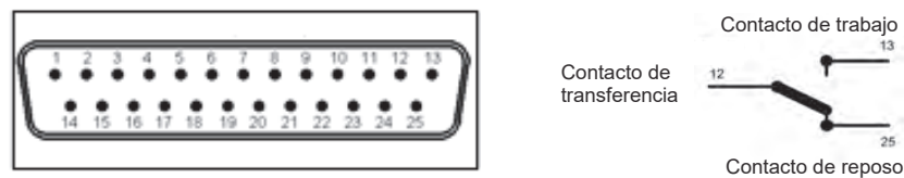
Figura: Ocupación de los zócalos Sub-D de 25 contactos - lado de soldadura
