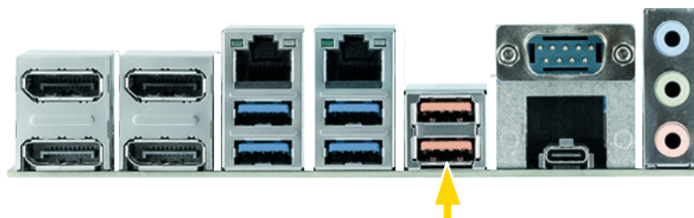
Figura 6: Conexiones USB
