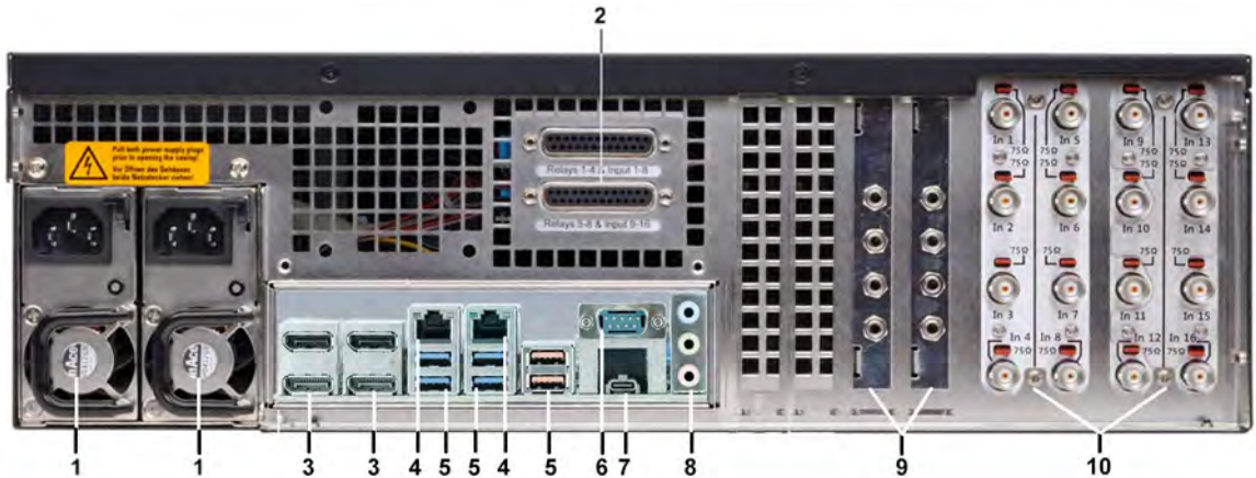
Abbildung 3: Rückansicht G-ST 6000+G3
