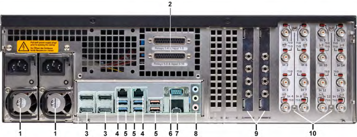
Figure 3: vue arrière G-ST 6000+ G3
