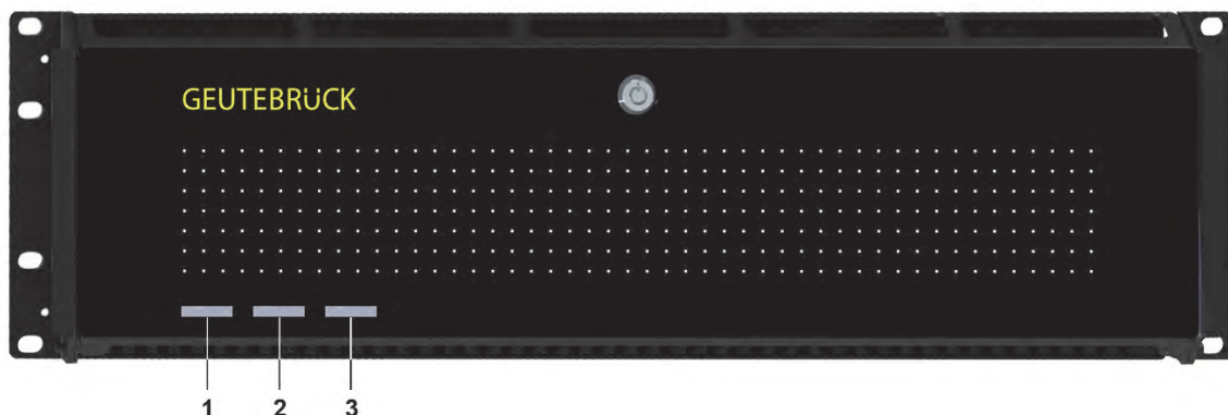
Abbildung 1: Frontansicht mit Blende
