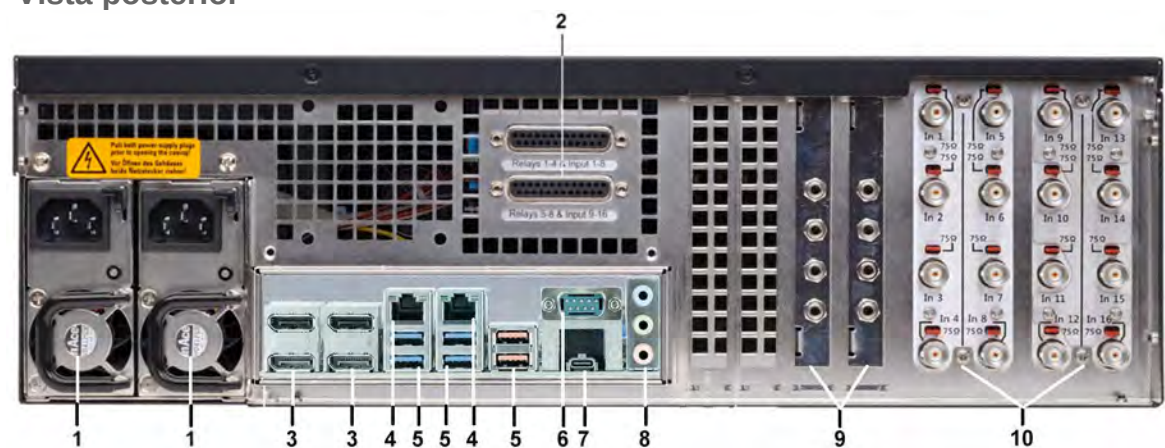
Figura 3: Vista posterior G-ST 6000+ G3
