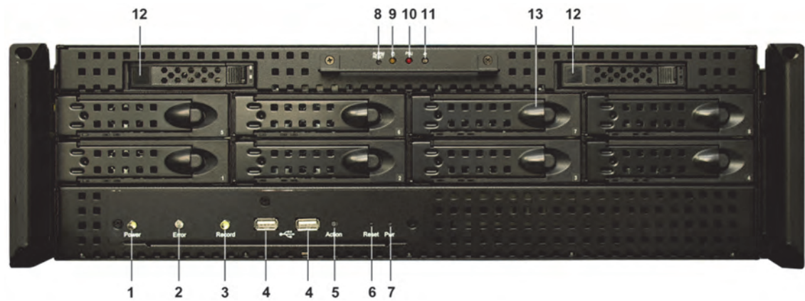
Figura 2: Vista frontal sin plate frontal
