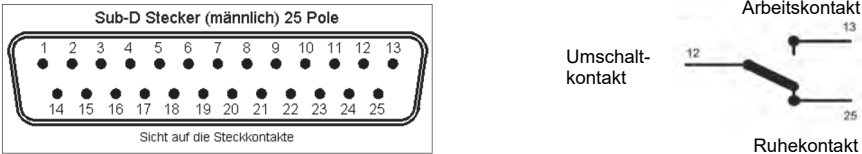
Abbildung 1: Belegung der 25-poligen Sub-D-Buchsen – lötseitig
