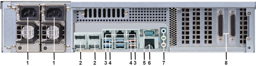
Figure : vue arrière G-ST 8000+G3/2U
