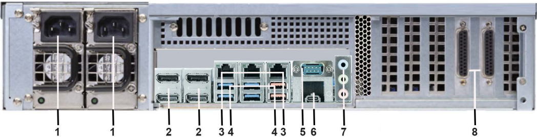
Figura: Vista posterior G-ST 8000+G3/2U
