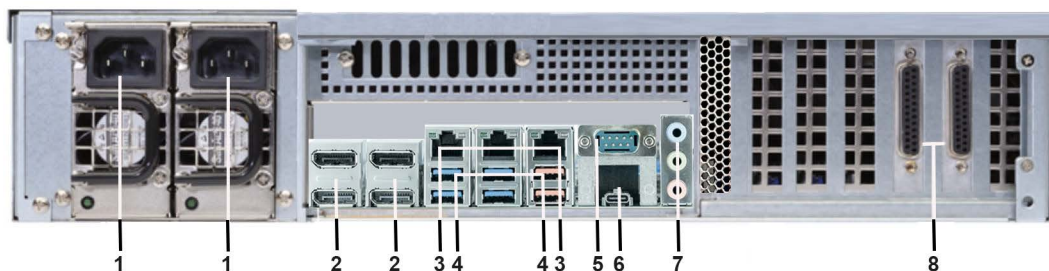
Abbildung: Rückansicht G-ST 8000+G3/2U
