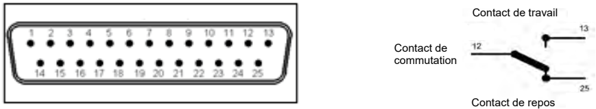
Figure : occupation des prises D-Sub à 25 bornes - côté soudure
